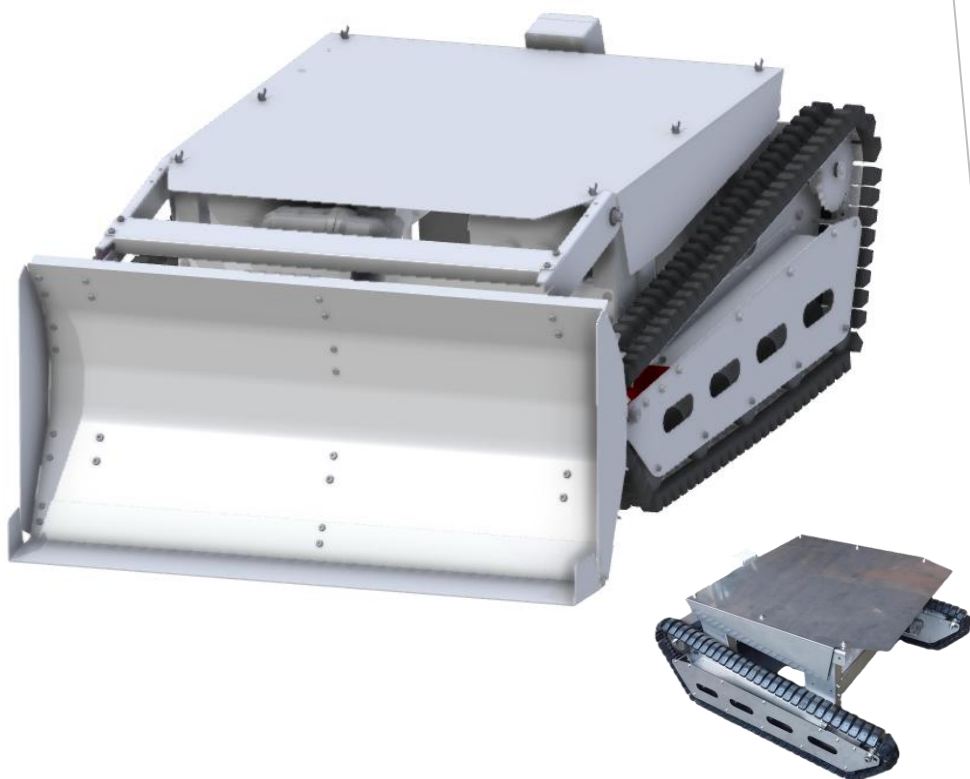
Uni Eベース（陸上ドローン）
